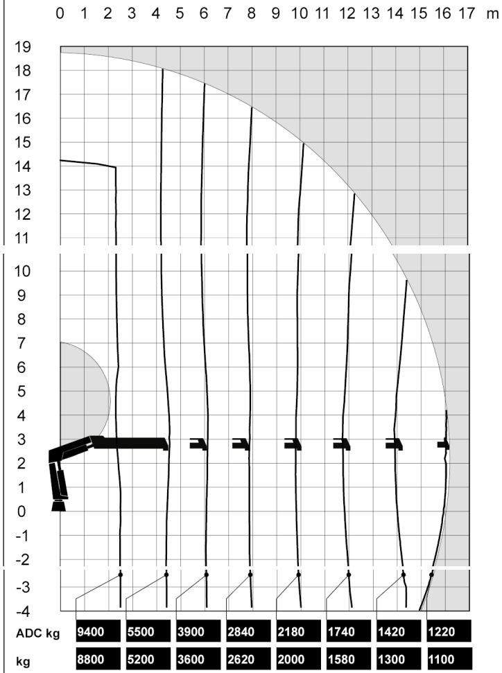
Belastungsdiagramm
