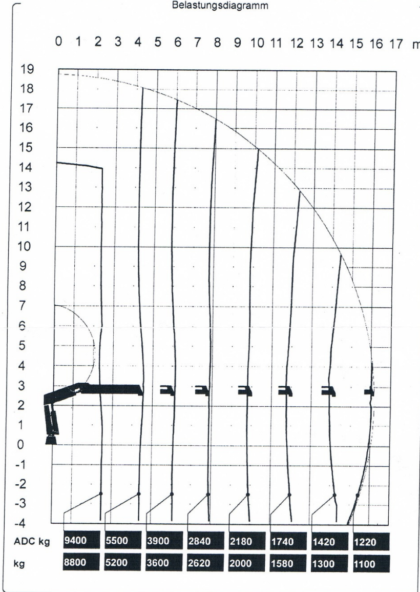
Belastungsdiagramm
